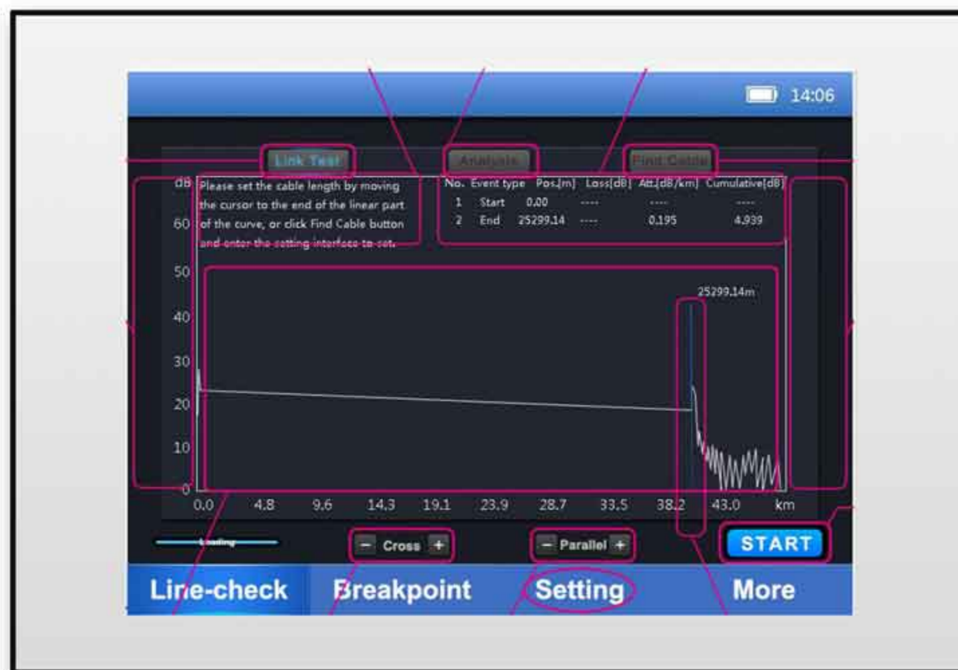
OTDR Function
